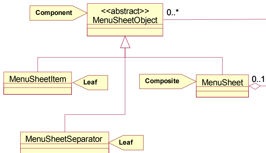
Abbildung 13 Das „Composite“ Muster angewandt auf Menüs.
