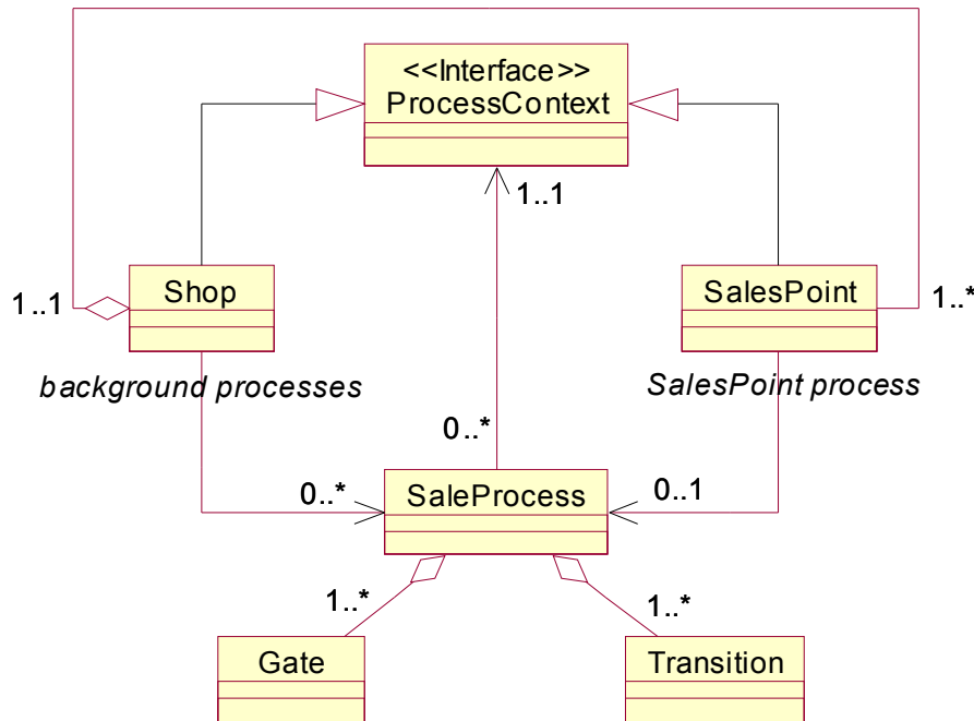
Abbildung 3 Prozesse können an Verkaufsständen und als Hintergrundprozesse laufen.
