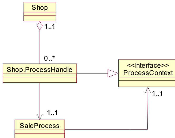
Abbildung 8 Tatsächliche Implementation des Ladens als Prozeßumgebung.
