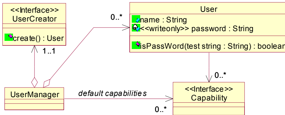
Abbildung 6 Benutzer haben Fähigkeiten und werden von Benutzermanagern verwaltet.
