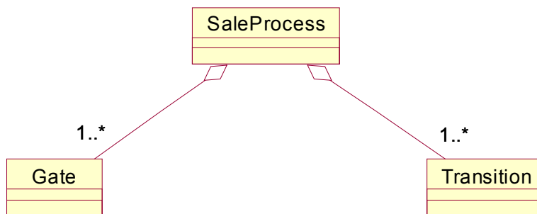
Abbildung 2 Ein Prozeß besteht aus Zuständen und Übergängen.
