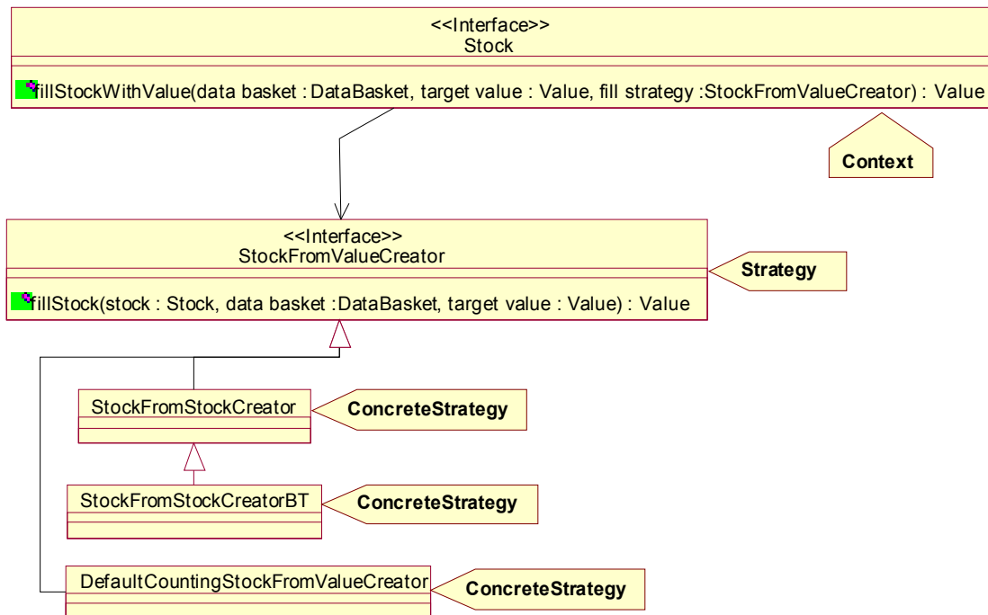
Abbildung 17 „Strategy“ Muster zum Stückeln von Werten und Auffüllen von Beständen.
