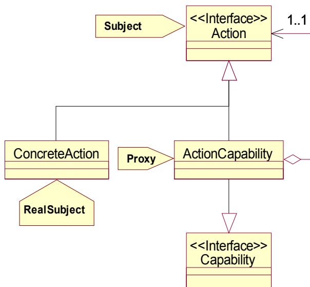
Abbildung 15 Eine Capability „bewacht“ eine Action .
