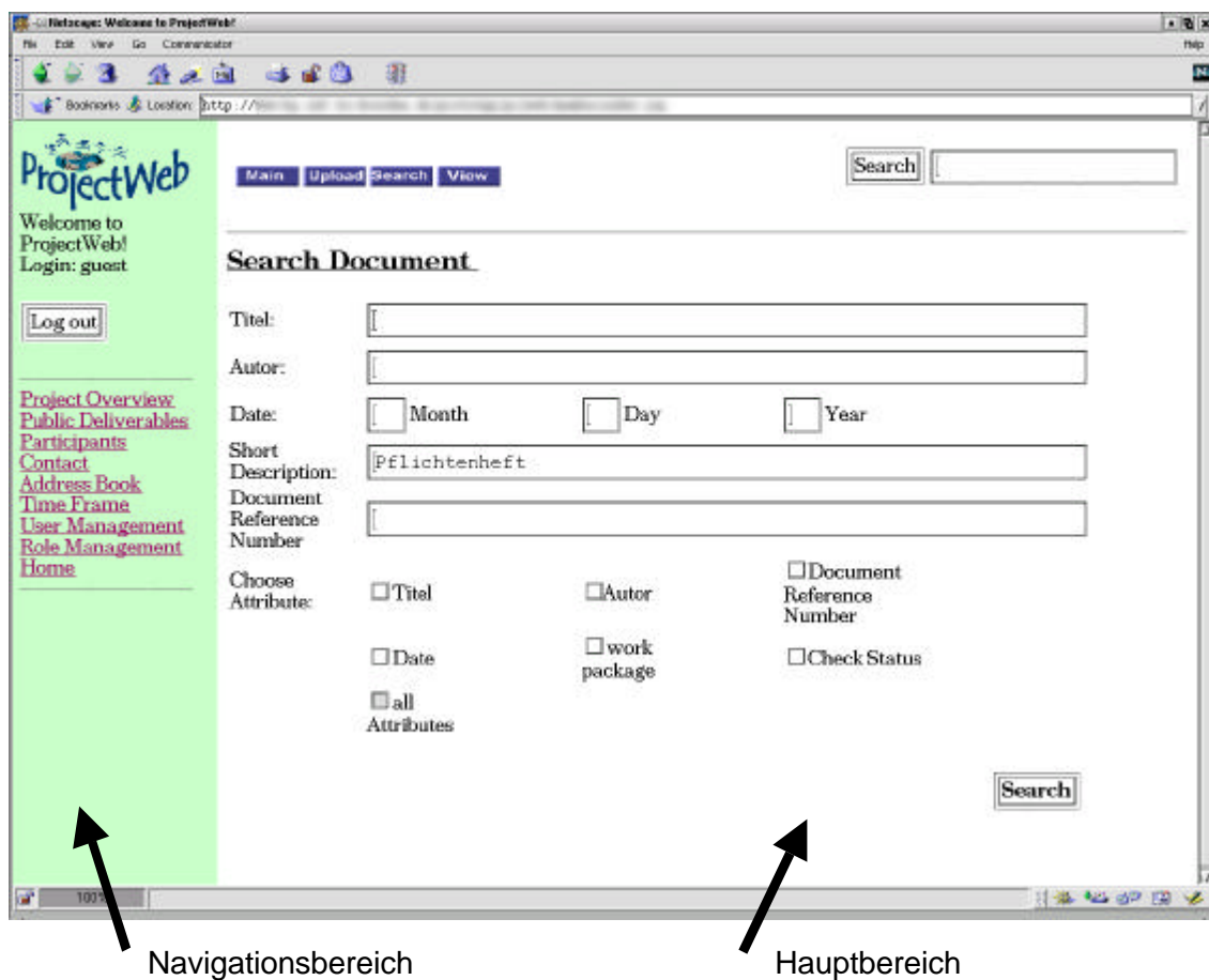
Abbildung 8: Benutzeroberfläche am Beispiel der globalen Suchfunktion nach bereits erfolgter Anmeldung am System
