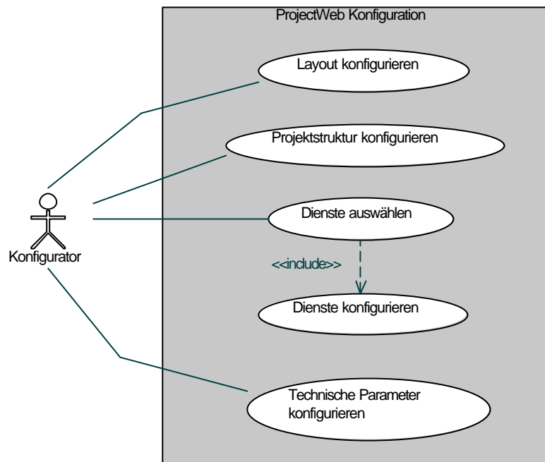
Abbildung 4: Anwendungsfall-Diagramm für die ProjectWeb-Konfiguration
