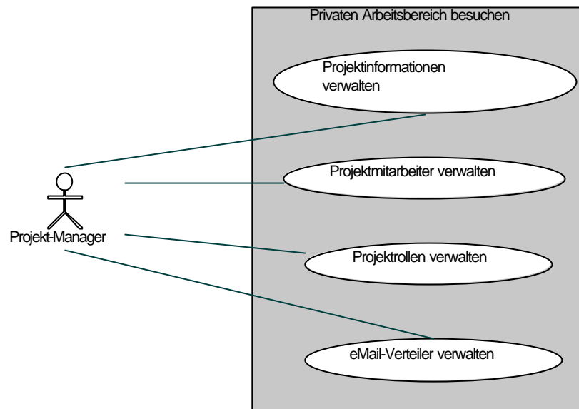
Abbildung 3: Anwendungsfall-Diagramm für den privaten Arbeitsbereich (2)
