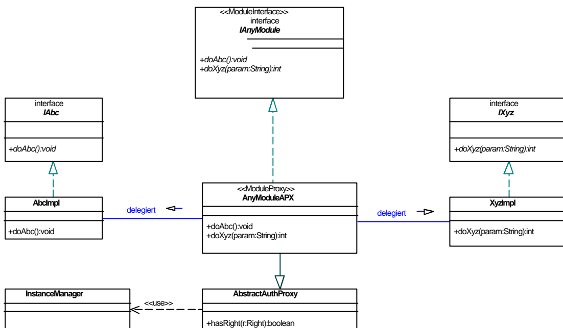
Abbildung 7: Rechteprüfung mit Module Proxy
