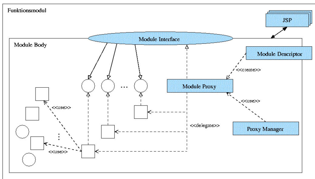
Abbildung 6: Aufbau eines Funktionsmoduls
