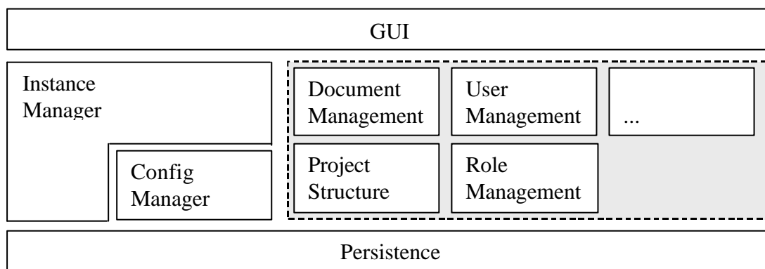
Abbildung 5: Grobarchitektur ProjectWeb – Blockdiagramm
