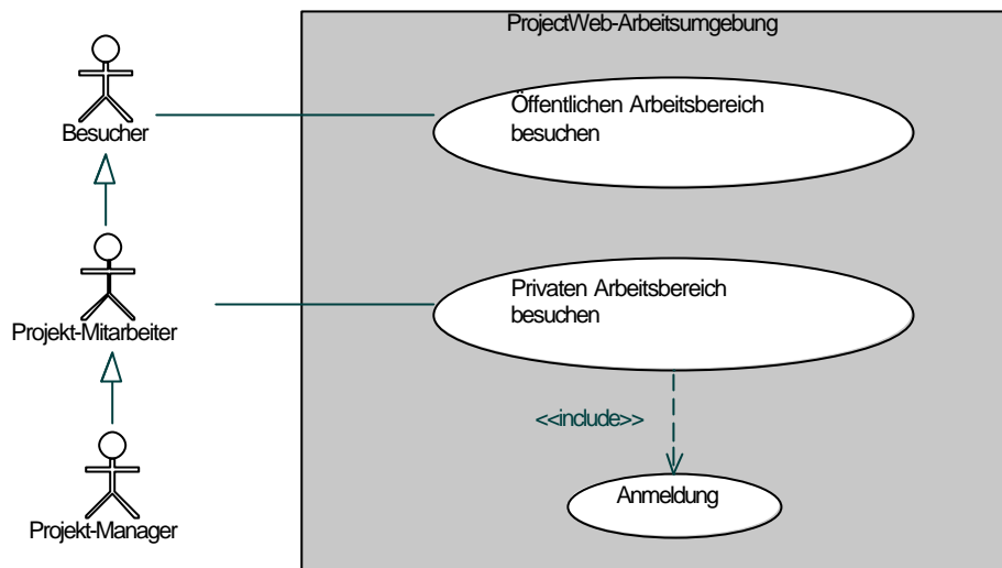
Abbildung 1: Anwendungsfall-Diagramm für eine ProjectWeb-Arbeitsumgebung
